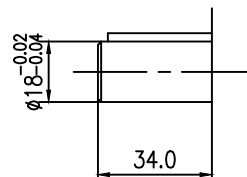
18轴平键
