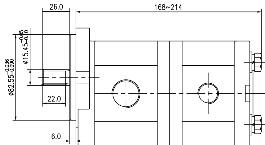
轴伸形式
