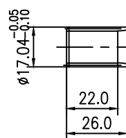
10齿渐开线花键
